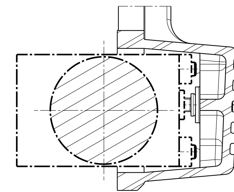
Schnitt G-G Maßstab: 1:1
